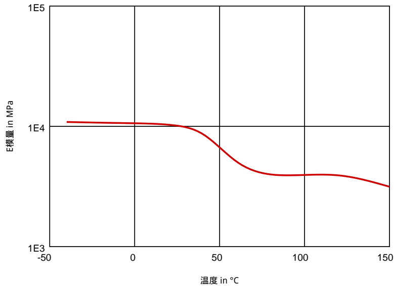
拉伸模量 - 温度(干)(measured on Zytel® 73G30HSL NC010)
