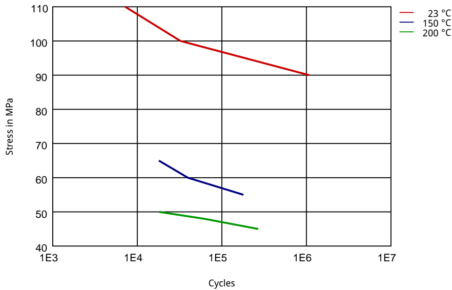
疲劳(Wöhler), 拉伸, 10Hz, R=0. mm(干)
