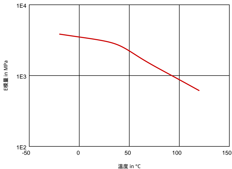
拉伸模量 - 温度 (measured on Delrin® 100 NC010)
